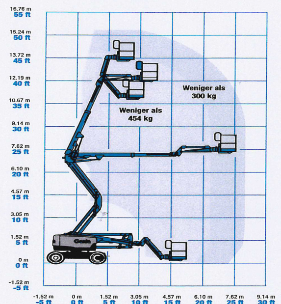
Arbeitsdiagramm Z-45XC
