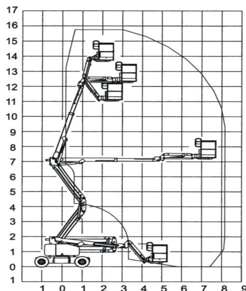
Reichweite – Modelle mit Korbausleger
